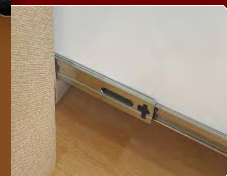
REFUERZO DE GUÍAS PARA CAJONES
